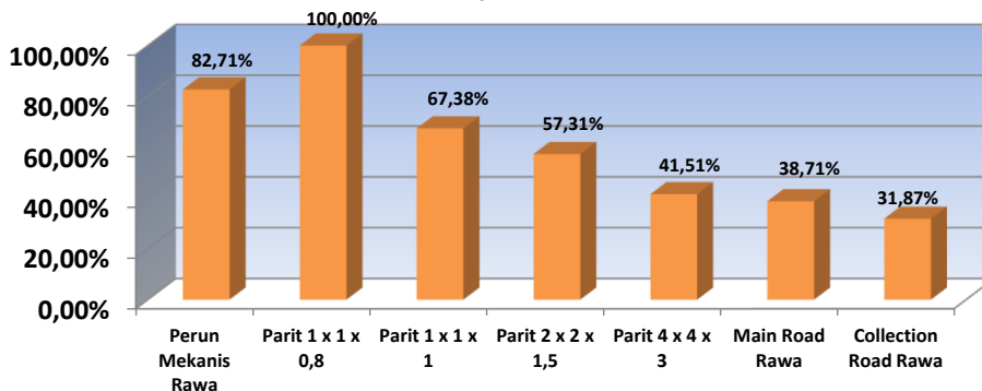
Pekerjaan Excavator
